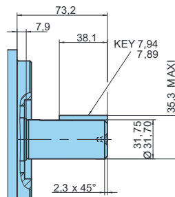
SHAFT CODE 2 (Keyed SAE)
